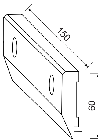
BRIDA SEGURETAT BRIDA SEGURIDAD SECURITY FLANGE
